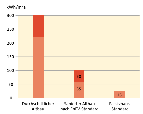
Abb. 4: Heizenergieverbrauch von Altbauten mit unterschiedlichem Standard (dunkelroter Bereich: Variationsbreite)
