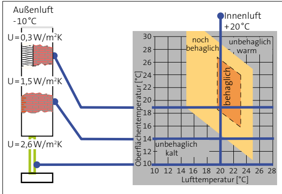
Abb. 1: Einfluss von Oberflächen- und Lufttemperatur auf die thermische Behaglichkeit
