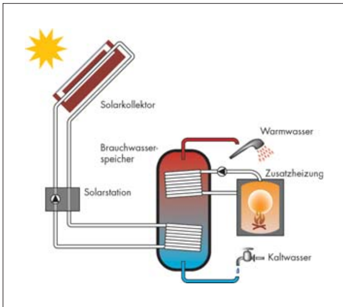
Abb. 3 Zweikreisssystem zur Warmwasserbereitung
