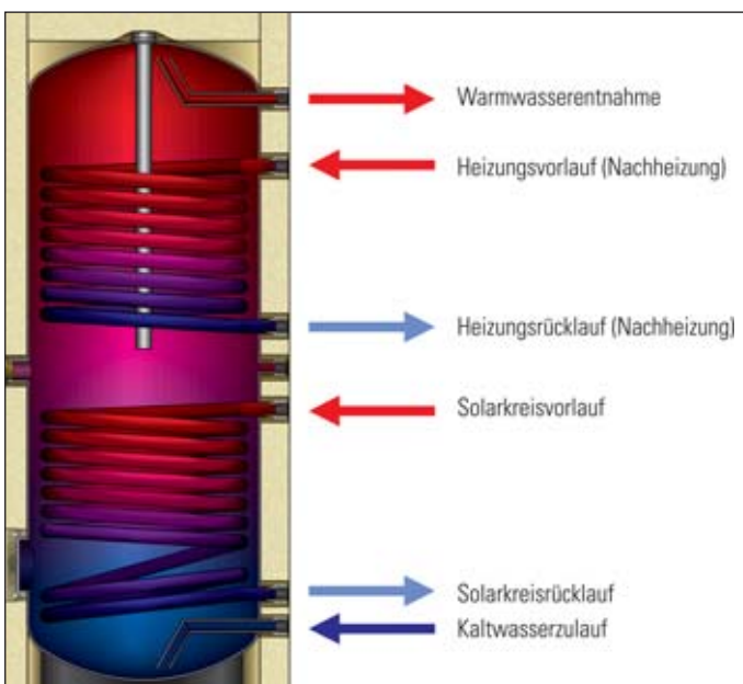
Abb. 7 Solarspeicher benötigen neben dem Wärmetauscher für die Heizung einen weiteren zur Einbindung des Kollektorkreises. (Quelle: Solarpraxis)
