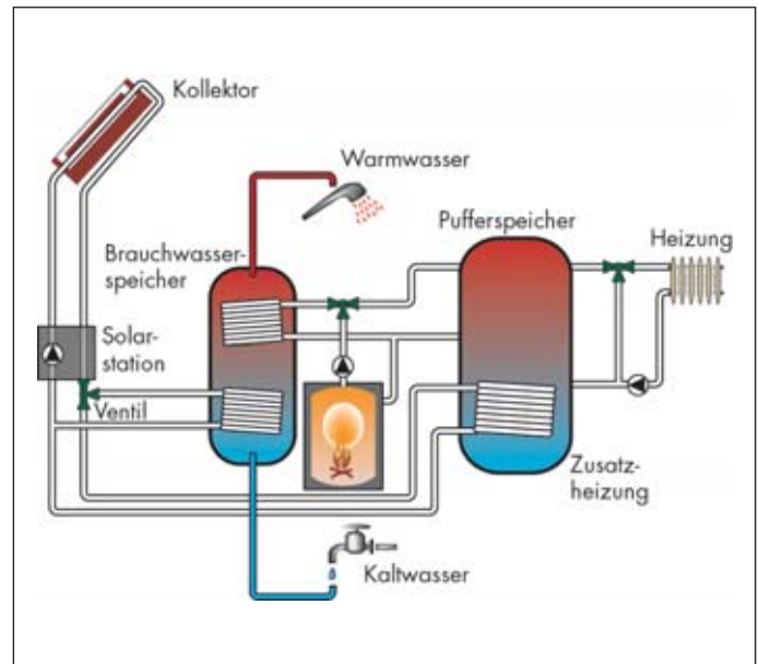
Abb. 4 Kombinierte solare Raum- und Warmwasserheizung mit Zweispeichersystem
