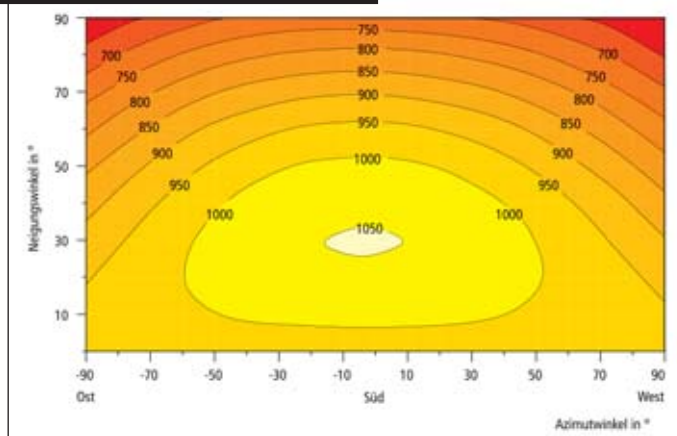
Abb. 8 Der Solarertrag ist abhängig von Ausrichtung und Neigung der Kollektorfläche. (Quelle: Solarpraxis)
