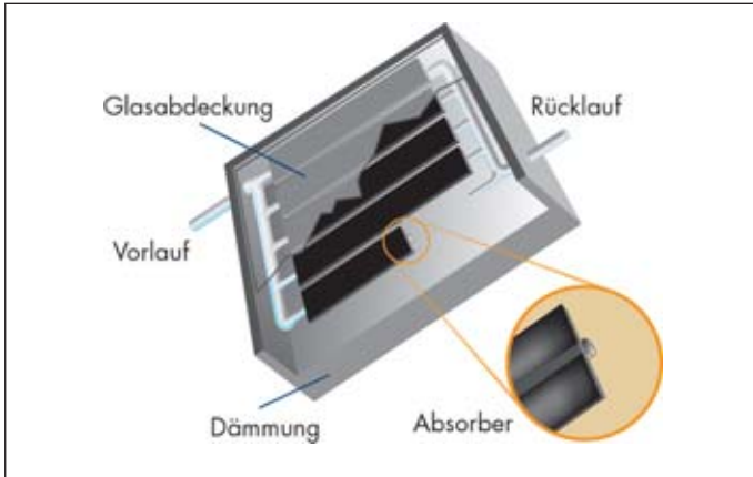
Abb. 5 Prinzipieller Aufbau eines Flachkollektors
