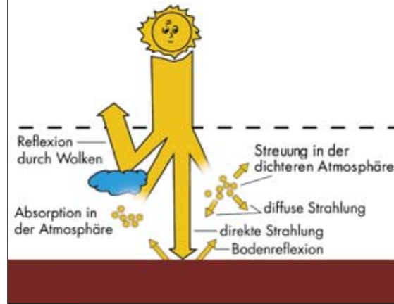
Abb. 2 Globalstrahlung besteht in Mitteleuropa je nach Jahreszeit zu 50–70% aus diffuser Strahlung.
