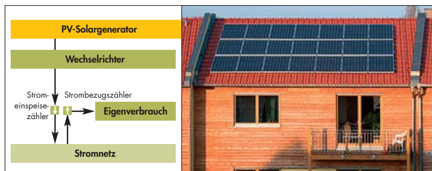
Abb. 7 Prinzipieller Aufbau einer netzgekoppelten Anlage. Nach dem Erneuerbare-Energien-Gesetz wird 20 Jahre der gesamte Solarstrom ins Netz eingespeist und kostendeckend vergütet, während der Eigenbedarf des Gebäudes normal aus dem Netz bezogen wird. (Quelle: BMU-Bilderdatenbank)
