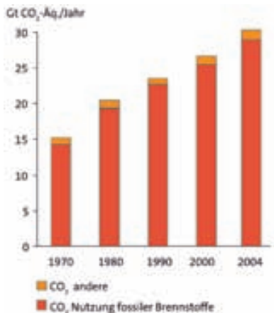
Abb. 3: Von fossiler Energieerzeugung verursachte Entwicklung der \text{CO}_2 -Konzentration in der Erdatmosphäre 1970 – 2004.
